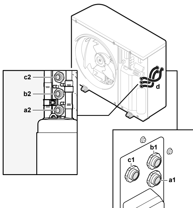
a1+a2 Napájecí kabel (lokálně dostupný díl) b1+b2 Propojovací kabel (lokálně dostupný díl)
